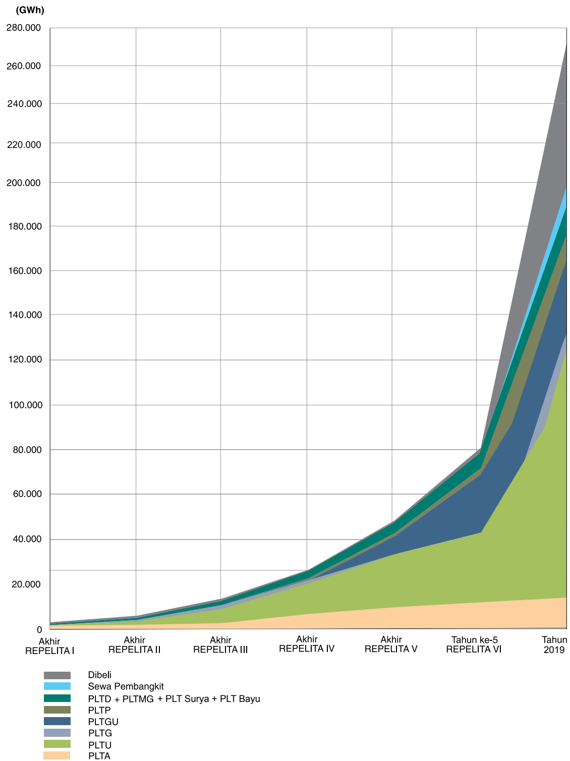
Grafik 12. Perkembangan Energi yang Diproduksi
