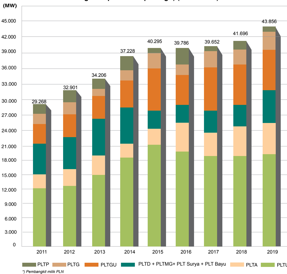
Grafik 7. Perkembangan Kapasitas Terpasang *) (2011 - 2019)
