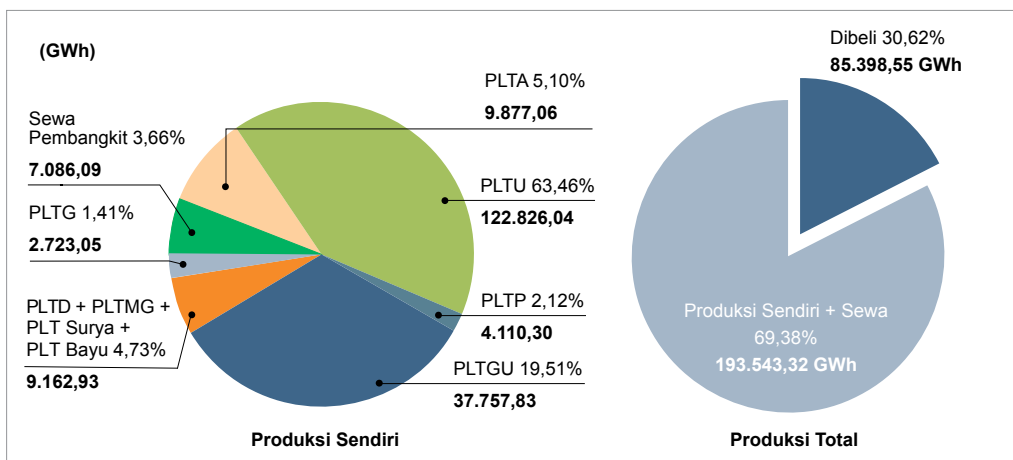
Grafik 4. Energi yang Diproduksi (2019)
